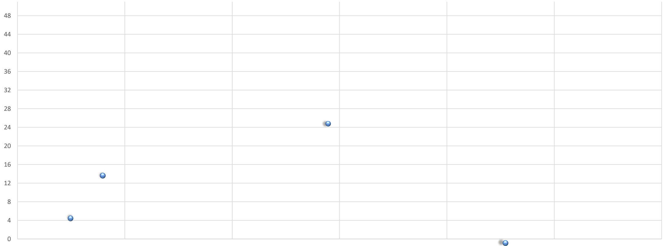
BMI
