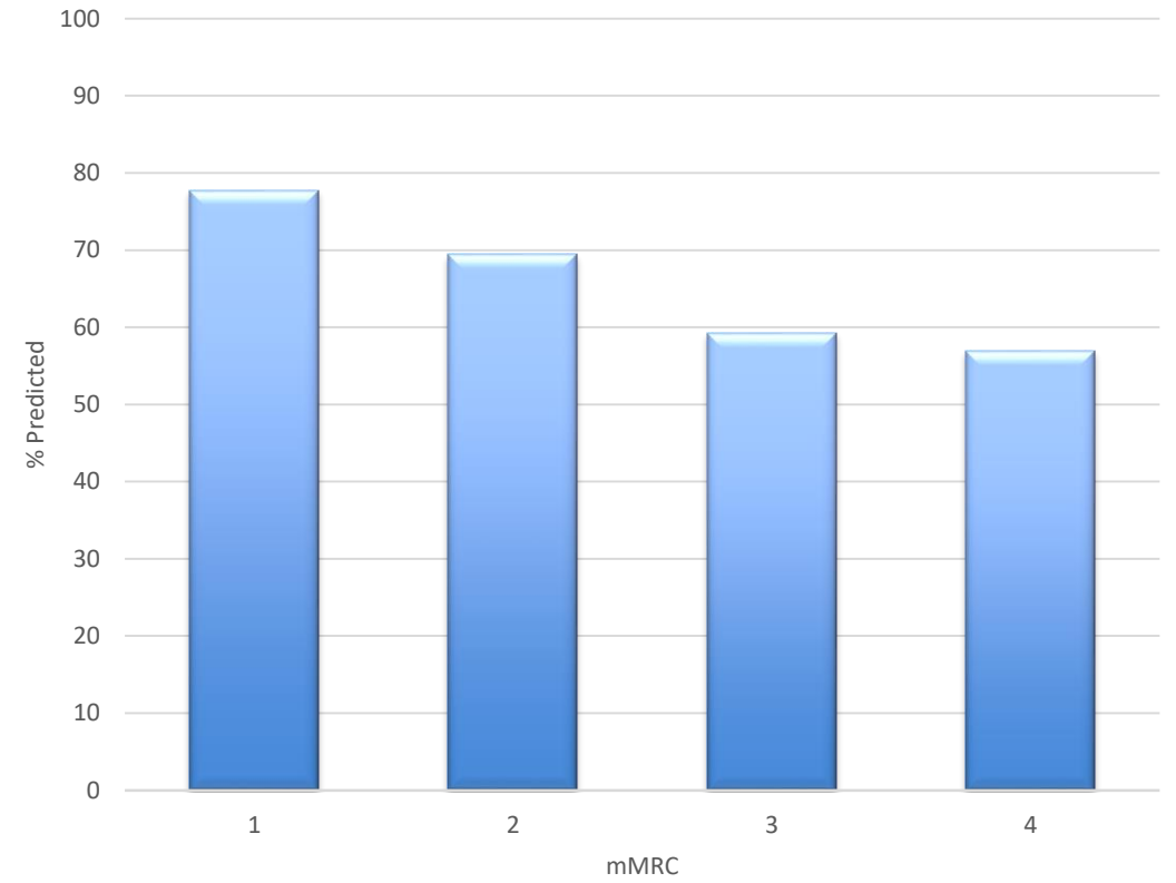
MIP
