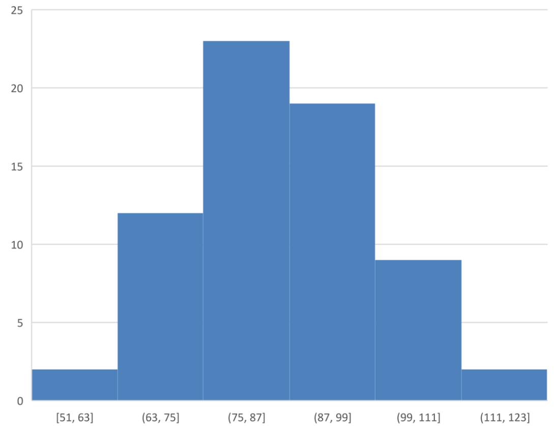
DLCO
