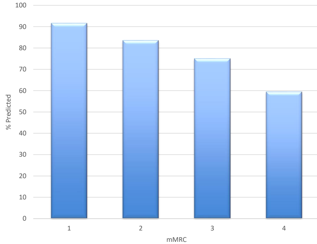
DLCO
