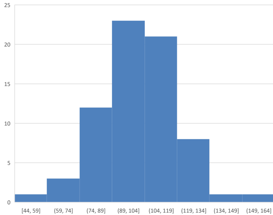
FEV1
